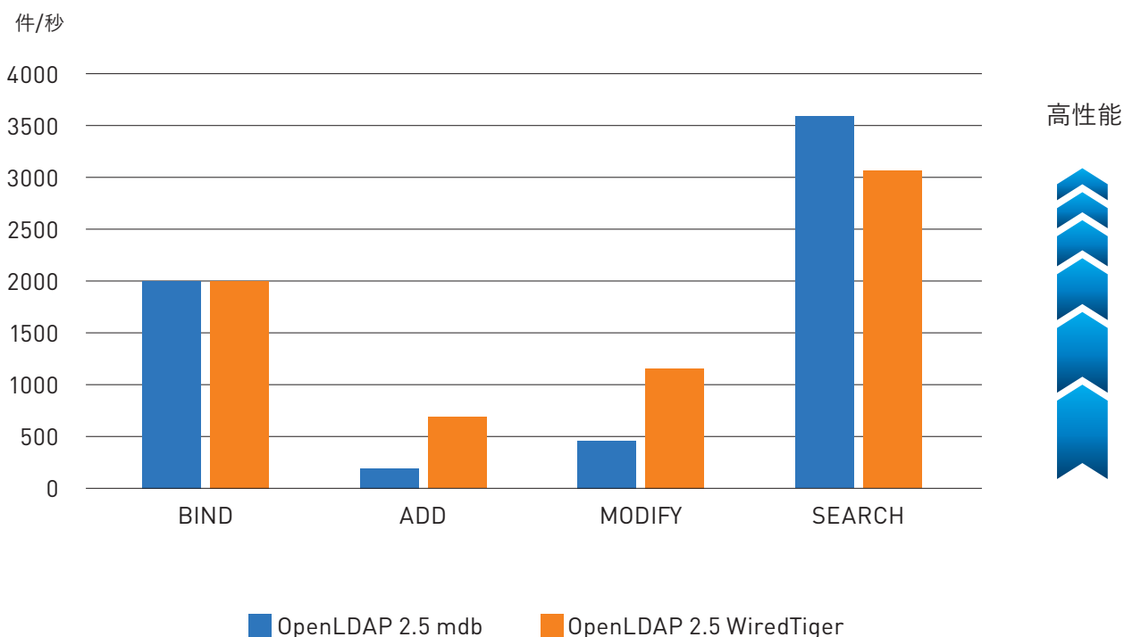
OSSTech OpenLDAP 2.5 性能測定値
